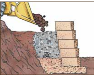
Diagram 5—Backfill
